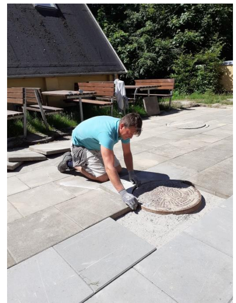
Flisetilpasning
